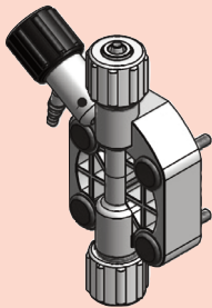
CORPO POMPA IN PVDF CON SPURGO MANUALE O AUTOMATICO
