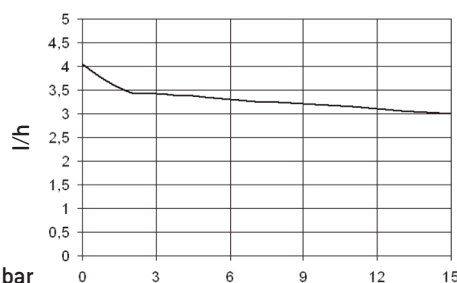
Variatione della portata massima in funzione della pressione dell'impianto
